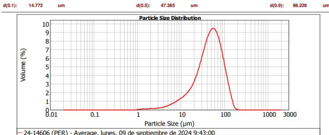
Figura 02. Granulometría Perlita P-05
