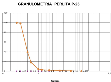
Figura 02. Granulometría Perlita P-25 (% Pasa acumulado)
