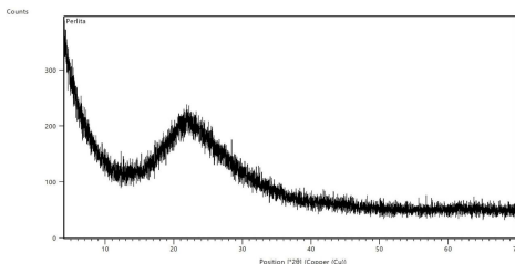
*Material 100% perlita* Figura 01. Difractograma
