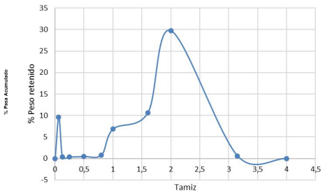
Figura 03. Granulometría Perlita P-25 (% Peso retenido)
